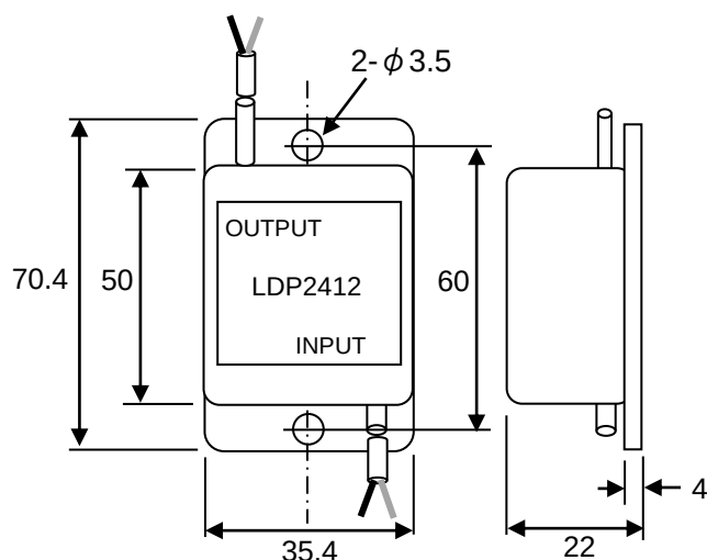
外形図
